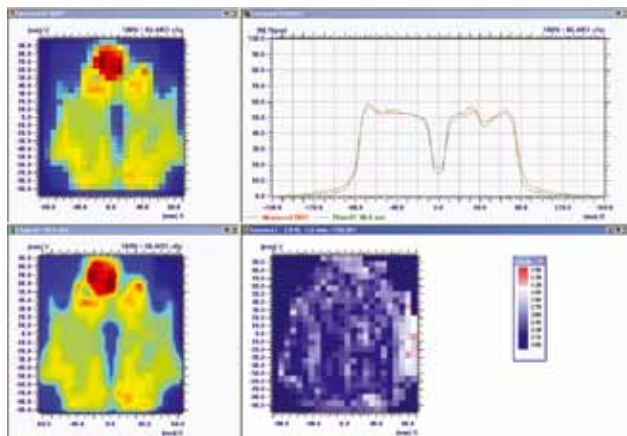
Slika 6. Primerjava med izmerjeno absorbirano dozo (levo zgoraj) in načrtovano dozo (levo spodaj) za anteroposteriorno usmerjeno polje.
